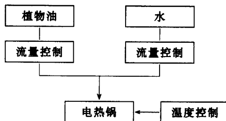
图2 油烟发生装置示意图
