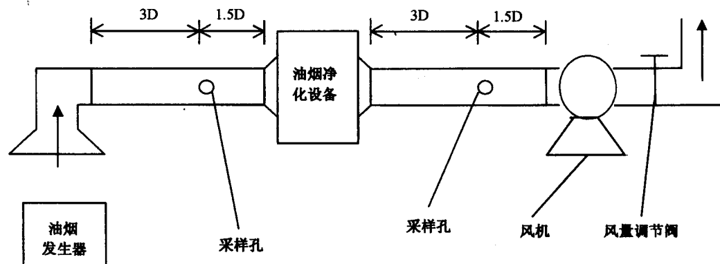
图 1 实验室油烟净化设备测试系统示意图
